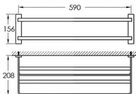
Towel Shelf FH8910
